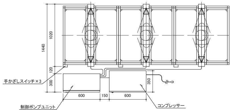
平面図
