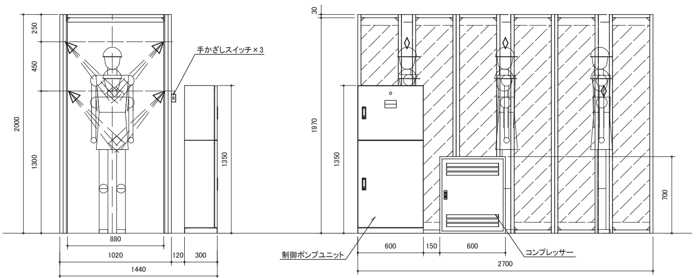
入口面図
