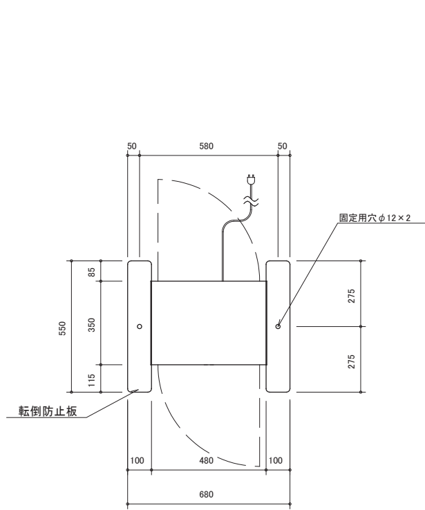
平面図
