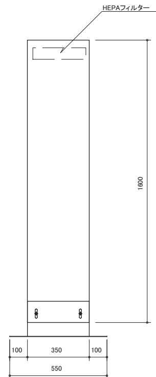
側面図
